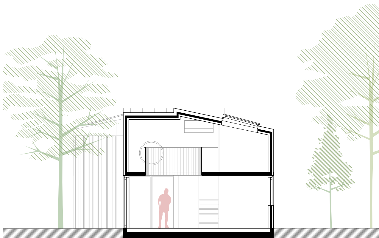
Schnitt durch das Atrium / Section through the atrium
