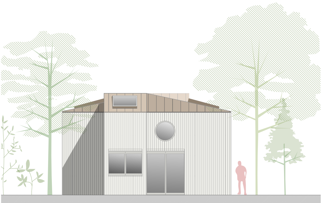
Ansicht / Elevation
