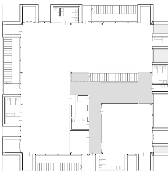
Obergeschoss / first floor
