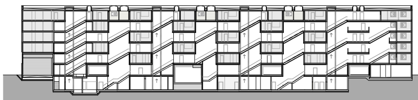
Längsschnitt straßenseitig Bauteil Ost/ Longitudinal section of building East
